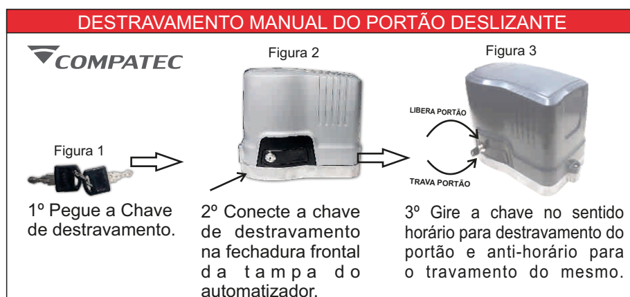
Figura 7: Destravamento manual do portão.
