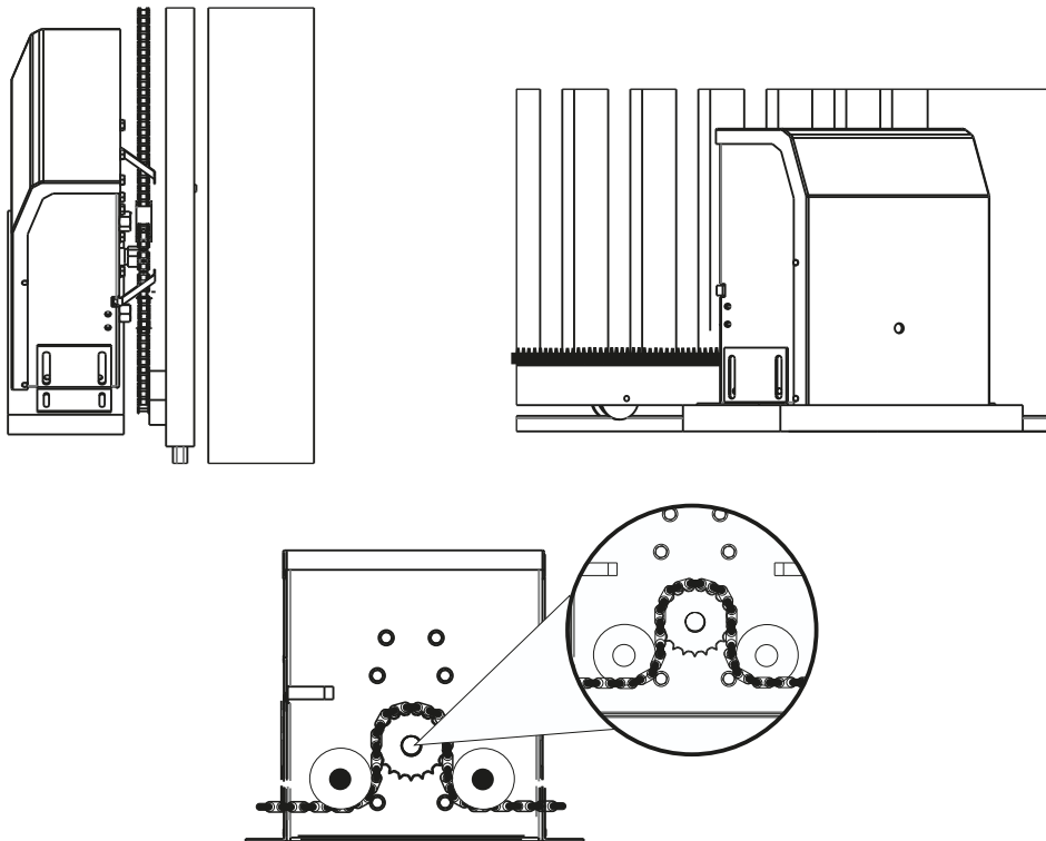
Figura 03: Transpassar a corrente conforme imagem e soldar no portão, com um ponto de solda, observando que a engrenagem se encaixe na corrente, para que ocorra a movimentação do portão no momento que o movimentador for acionado.
