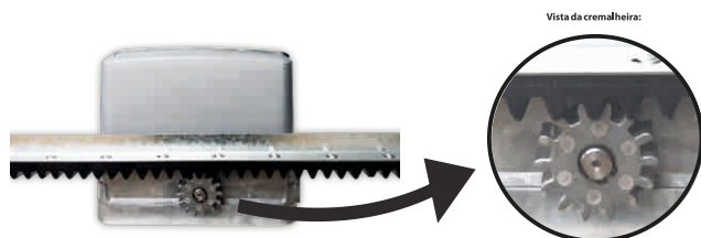
Figura 3: Vista del ajuste de la corona del automatizador corredizo na cremalleira listo para usar.
