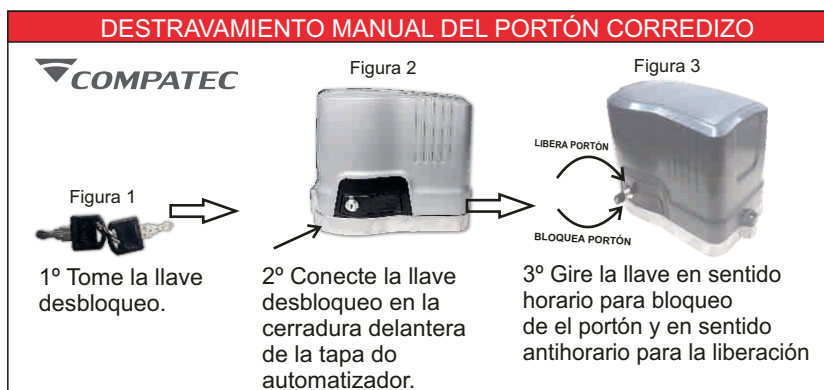
Figura 7: Destravamiento manual del portón.
